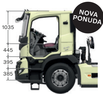
NISKA DNEVNA KABINA
