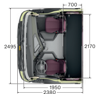
KABINA ZA POSADU
